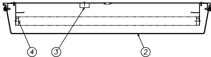
B-B断面図
